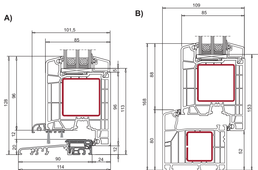
Haustür Flügel Nr. 7033 116 mm thermisch getrennte HT-Schwelle Nr. 8520 90 mm Wetterschenkel Ev1
