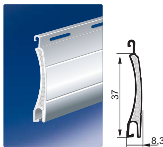
Mini-Profil AP.S/37
