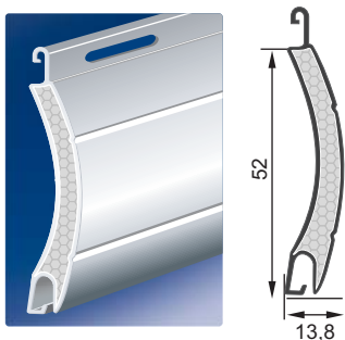
Maxi-Profil AP.S/52
