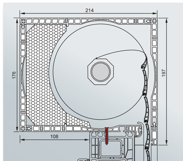
18er Aufsatzelement
