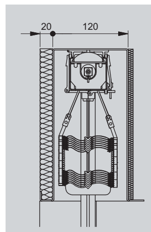
Modulo P einputzbar mit 20 mm Hinterdämmung (auch bei sicht- barem P-System möglich)
