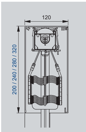
Modulo P sichtbare Blende (stranggepresst)
