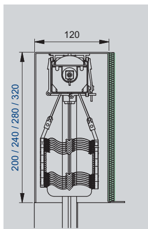
Modulo P einputzbar (Blende gekantet)
