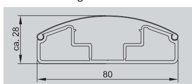
Lamelle GL 80 gebördelt
